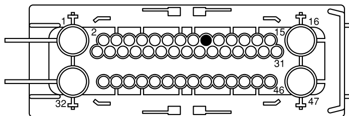
メスコネクタを配線側から見た図
