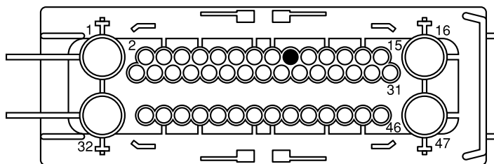
メスコネクターを配線側から見た図
