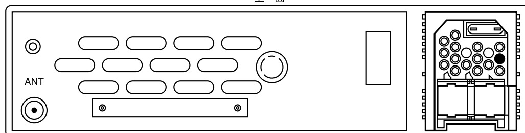
純正カセットデッキを上図矢印方向から見た図
