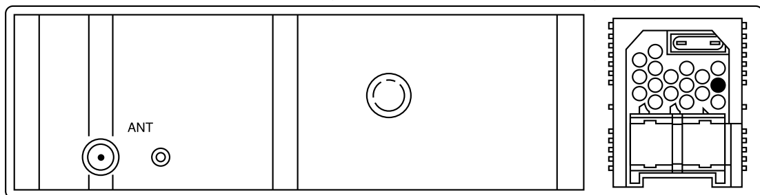
コネクタを配線側から見た図
