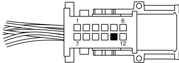
メスコネクターを端子側から見た図
