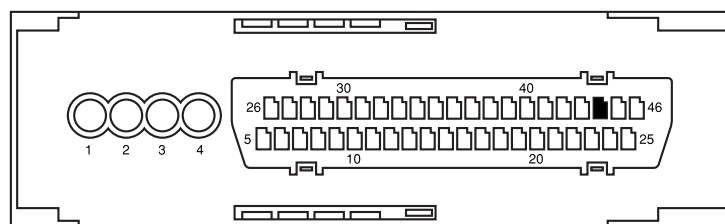
メスコネクタを配線側から見た図
