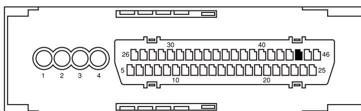
メスコネクターを配線側から見た図
