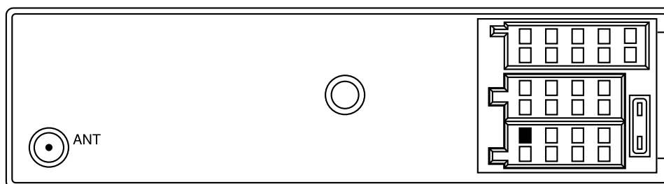
純正カセットデッキを上図矢印方向から見た図
