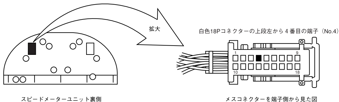
スピードメーターユニット裏側
