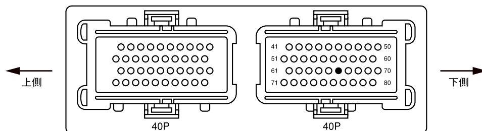
パワートレーンコントロールモジュールのコネクタを配線側から見た図
