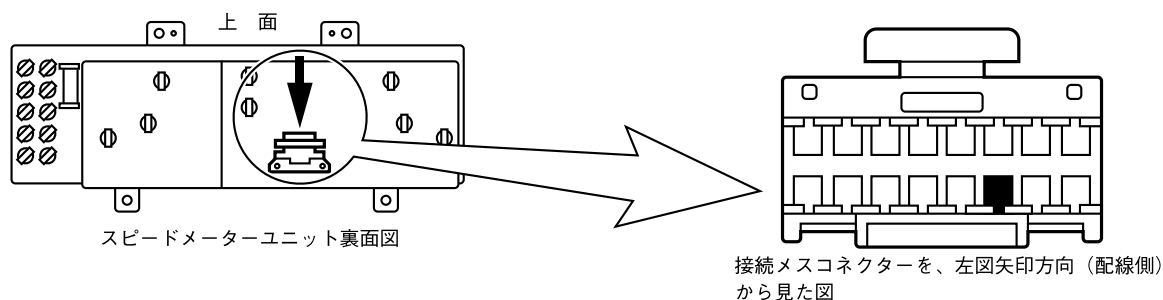
スピードメーターユニット裏面、接続コネクター (黒色16P)
