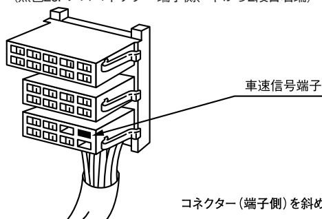
純正デッキ接続コネクタ (黒色26Pメスコネクタ端子側、下から2段目右端)
