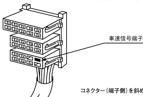
カセットデッキ接続コネクタ (黒色26Pメスコネクタ端子側、下から2段目右端)
