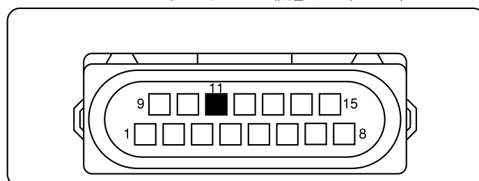
メスコネクターを配線側から見た図
