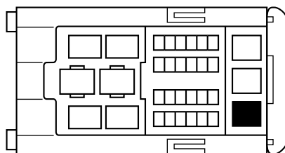
オスコネクタを配線側から見た図
